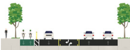
제안된 자전거 길의 단면도
